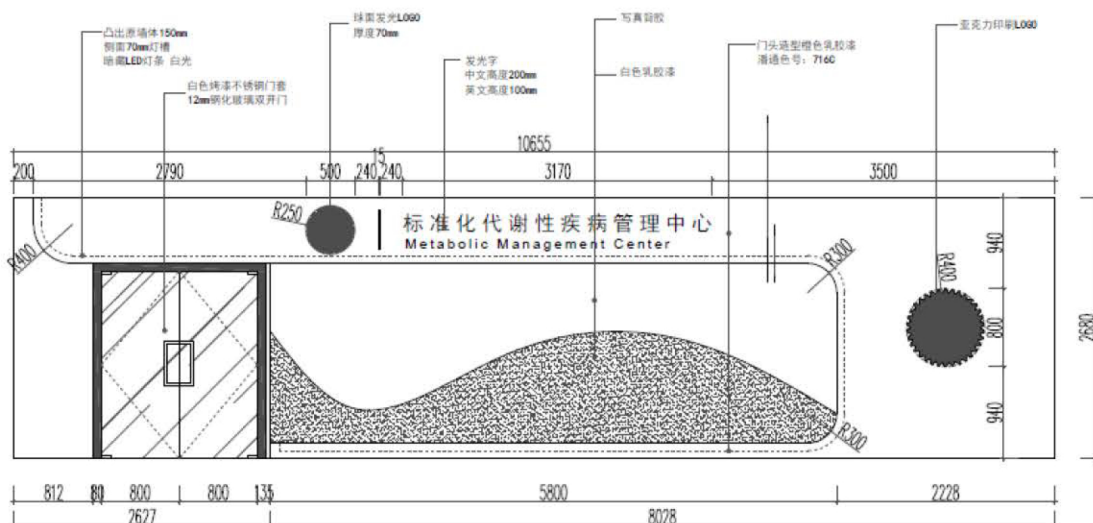
外部形象墙尺寸
