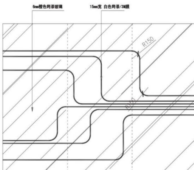
内部形象墙二 尺寸和标准工艺
