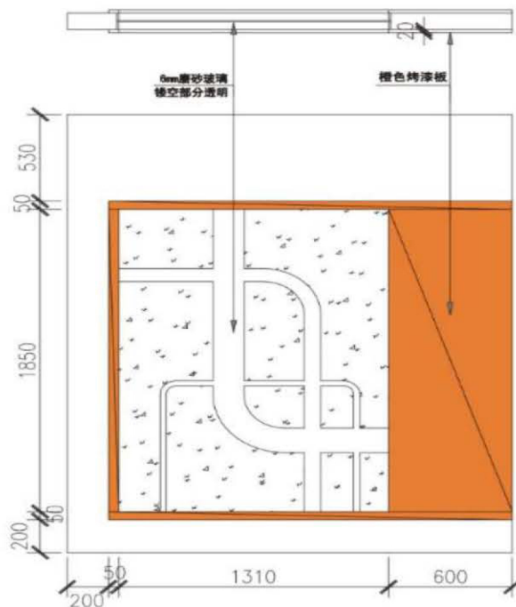
隔断一 尺寸和标准工艺
