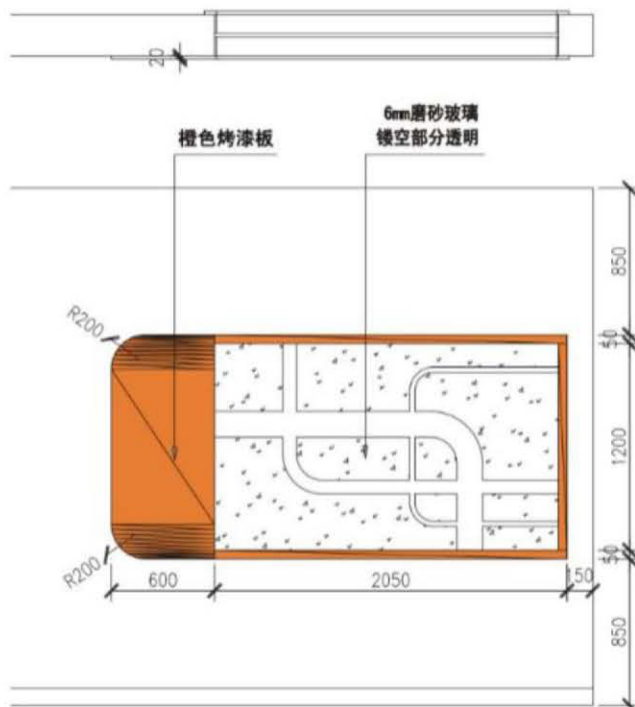
隔断二 尺寸和标准工艺
