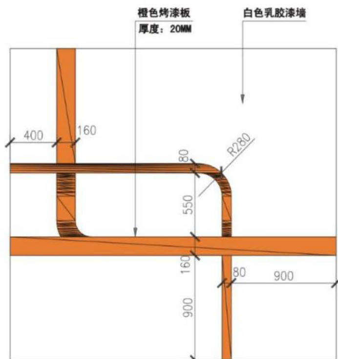
内部形象墙一 尺寸和标准工艺
